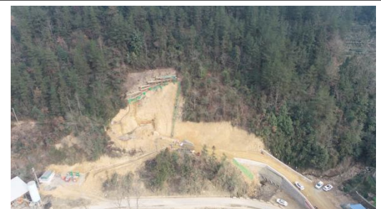
交通洞出口洞脸开挖支护
